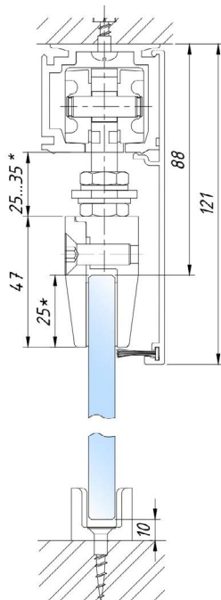
схема крепления к потолку
