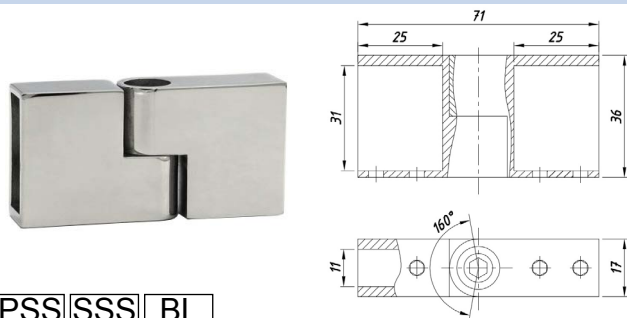
SF-2641 Соединитель труба-труба произвольный угол
