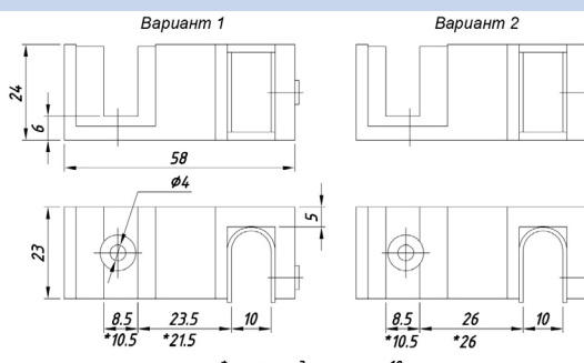
SF-505-D Нижняя направляющая
