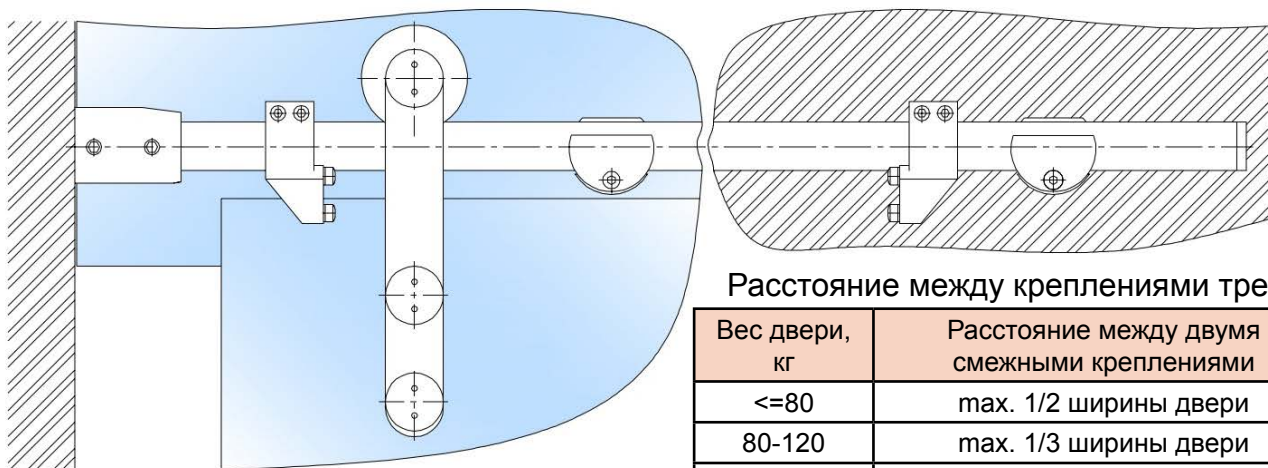
Расчет длины трека
