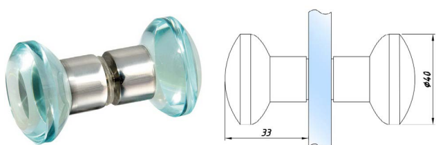
SF-686 Ручка-кноб стеклянная круглая
