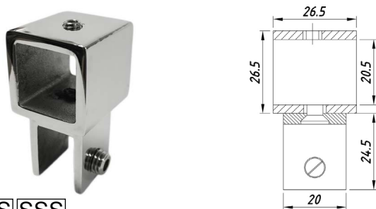
SF-2686 Соединитель труба-труба 90°
