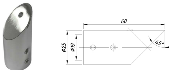
SF-945 Соединитель труба-стена 45°
