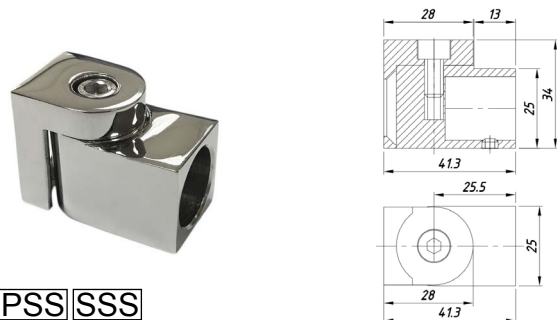
SF-914 Соединитель труба-стекло сквозной
