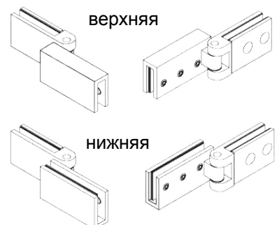
положение «открыто»
