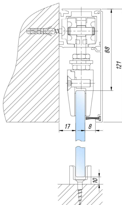
схема крепления к стене
