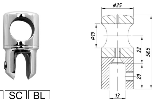
SF-914B Соединитель труба-стекло сквозной удлинённый
