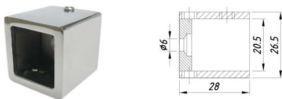
SF-2685 Соединитель труба-стена
