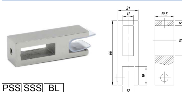
SF-2639 Соединитель труба-стекло торцевой
