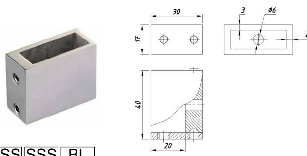
SF-2637 Соединитель труба-стена
