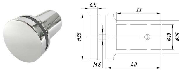
SF-906 Соединитель труба-стекло торцевой
