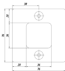
SF-71-59 Ручка-кноб прямоугольная
