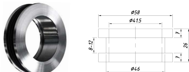
SF-71-39L Ручка-кноб таблетка сквозная
