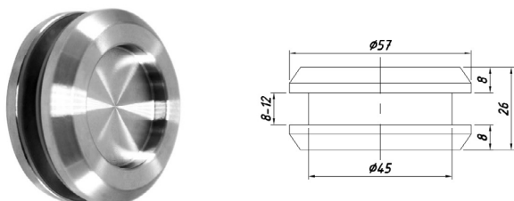
SF-71-29L Ручка-кноб таблетка большая
