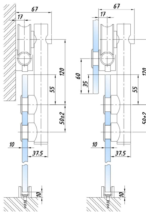
Каретка цилиндрическая
