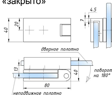
положение «закрыто»
