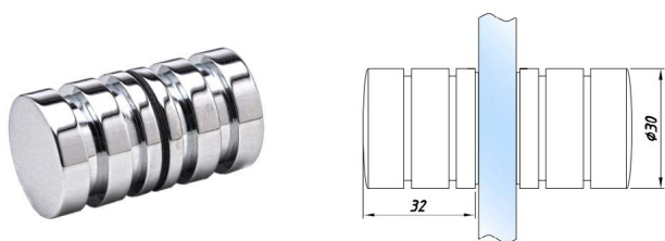
SF-71-24 Ручка-кноб
