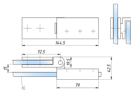
положение «открыто»
