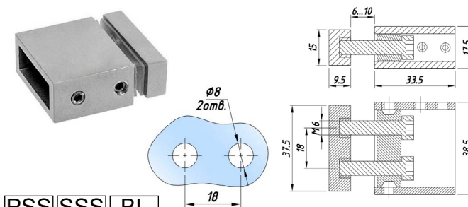
SF-505-D Нижняя направляющая
