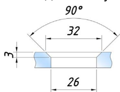
Каретка плоская
