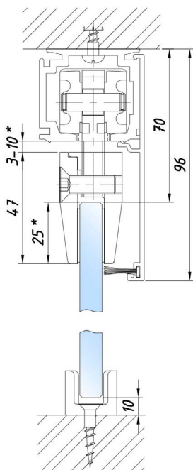
схема крепления к потолку
