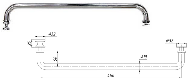
SF-621 Ручка с полотенцесушителем
