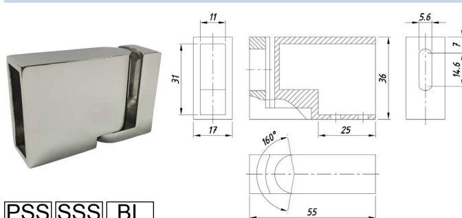
SF-2642 Соединитель труба-стена произвольный угол
