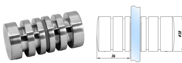
SF-71-24L Ручка-кноб большая
