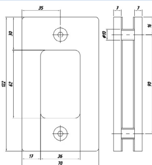
SF-71-59 Ручка-кноб прямоугольная
