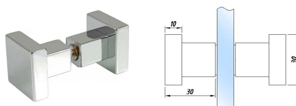
SF-684 Ручка-кноб квадратная
