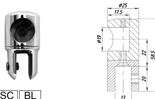
SF-906 Соединитель труба-стекло торцевой
