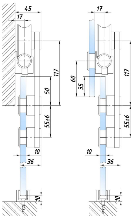
Каретка плоская
