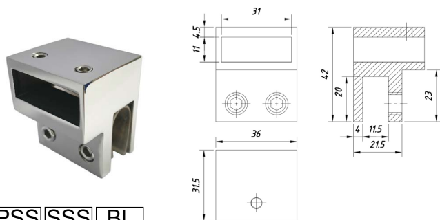
SF-2632 Соединитель труба-стекло глухой
