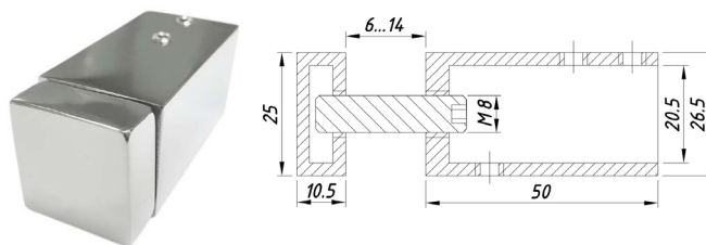
SF-2692-1 Соединитель труба-стекло торцевой
