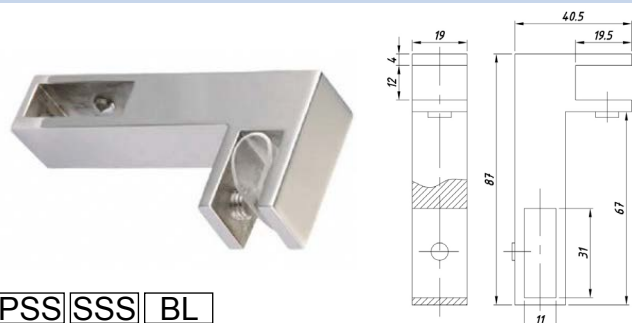
SF-9009-2 Коннектор труба-стекло
