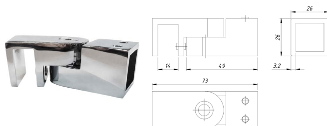
SF-2695 Соединитель труба-стекло
