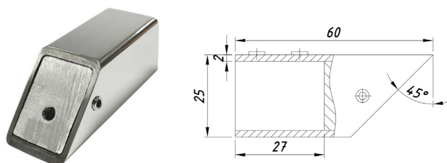
SF-2645 Соединитель труба-стена 45°
