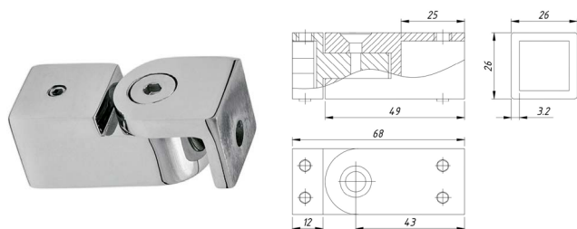
SF-2690 Соединитель труба-стена
