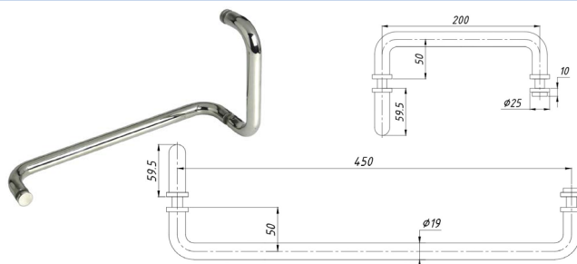
SF-626 Ручка с полотенцесушителем
