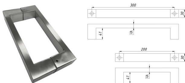
SF-2736 Ручка прямоугольная
