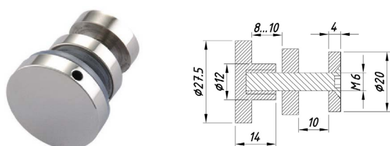
SF-9009-2 Коннектор труба-стекло
