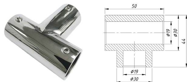
SF-902 Соединитель Т-образный
