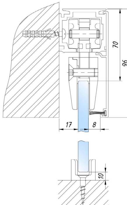
схема крепления к стене
