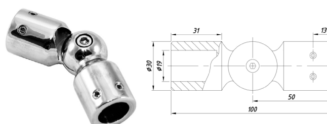
SF-915 Соединитель с произвольным углом
